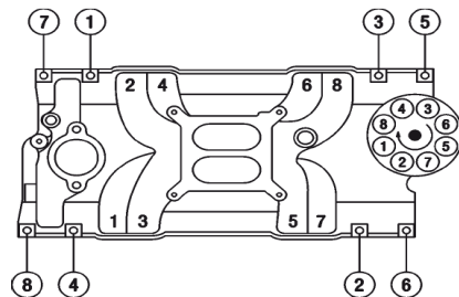
ORDRE D'ALLUMAGE 1-8-4-3-6-5-7-2
